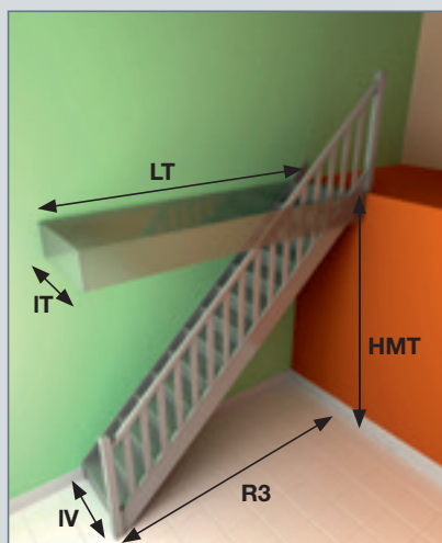
Escalier droit
